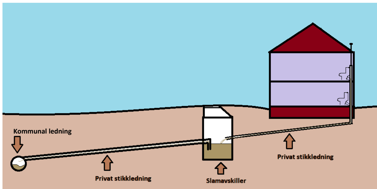
Prinsippkisse 1: Slamavskiller før tilknytning kommunal avløpsledning
