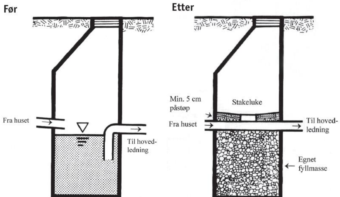
Prinsippskisse 2. slamavskiller før og etter utkobling.
