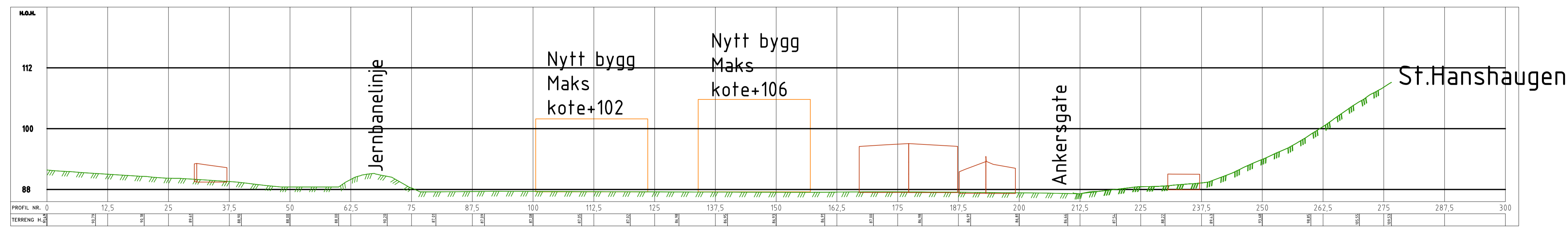
Lengdesnitt Vest-øst
