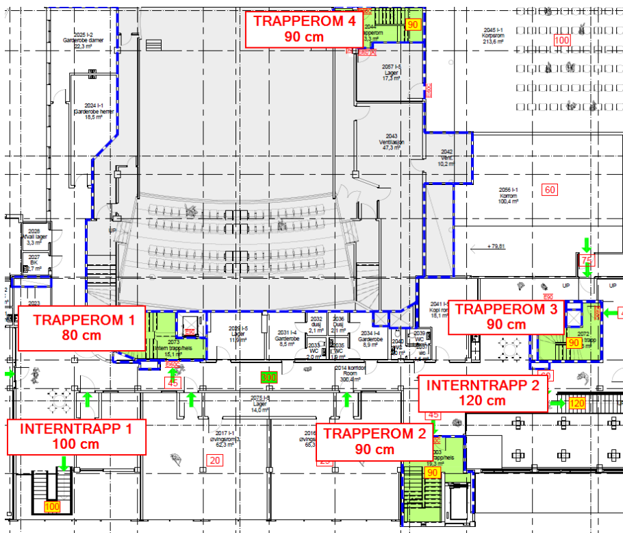
Figur 6-1. Utsnitt av branntegning for plan 1 for å illustrere fordeling og nummerering av trapperom og interntrepper.
