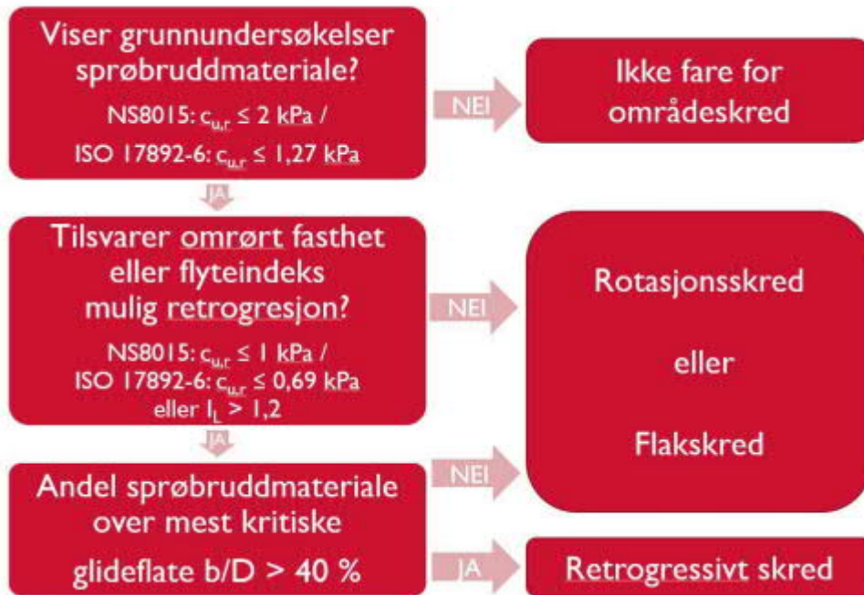
Figur 10: Flytskjema for vurdering av aktuell skredmekanisme, hentet fra NVEs veileder 1/2019.
