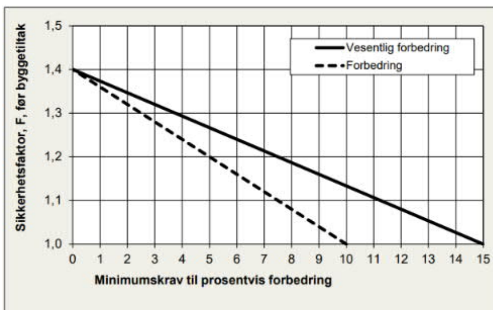
Figur 7: Krav til prosentvis forbedring av sikkerhetsfaktor, F_{\phi} og F_{cu} .
