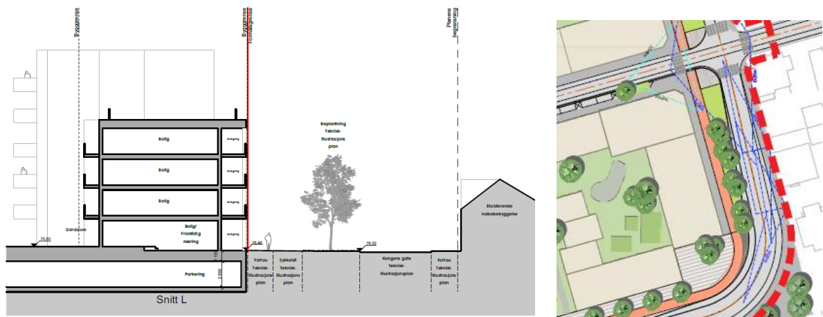
Figur 19 - Snitt K gjennom bebyggelse mot Kongens gate og utsnitt gateutforming i teknisk illustrasjonsplan.
