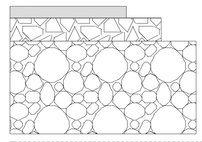
Prinsippskisse av vegoppbygning
