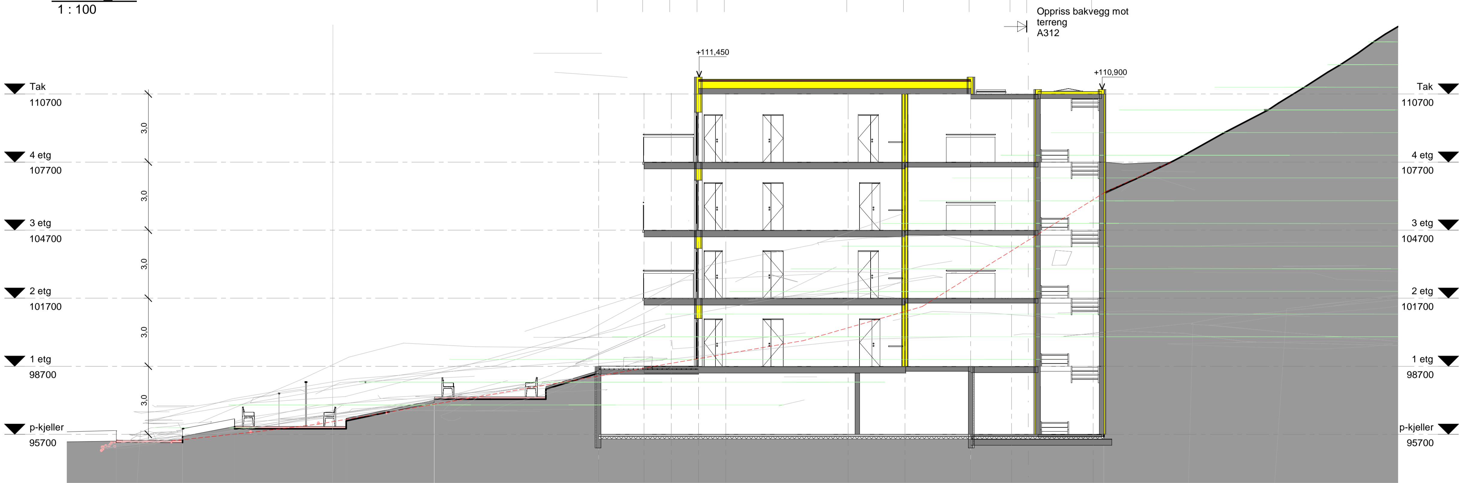
Snitt B B 1 : 100
