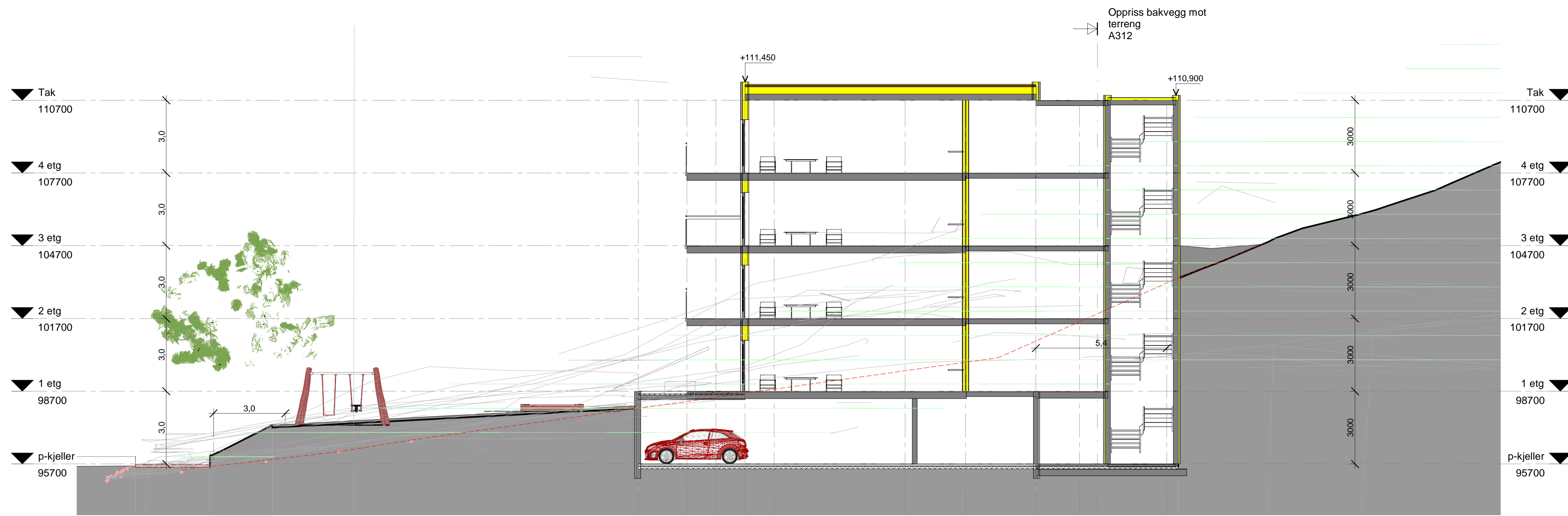
Snitt A A 1 : 100
