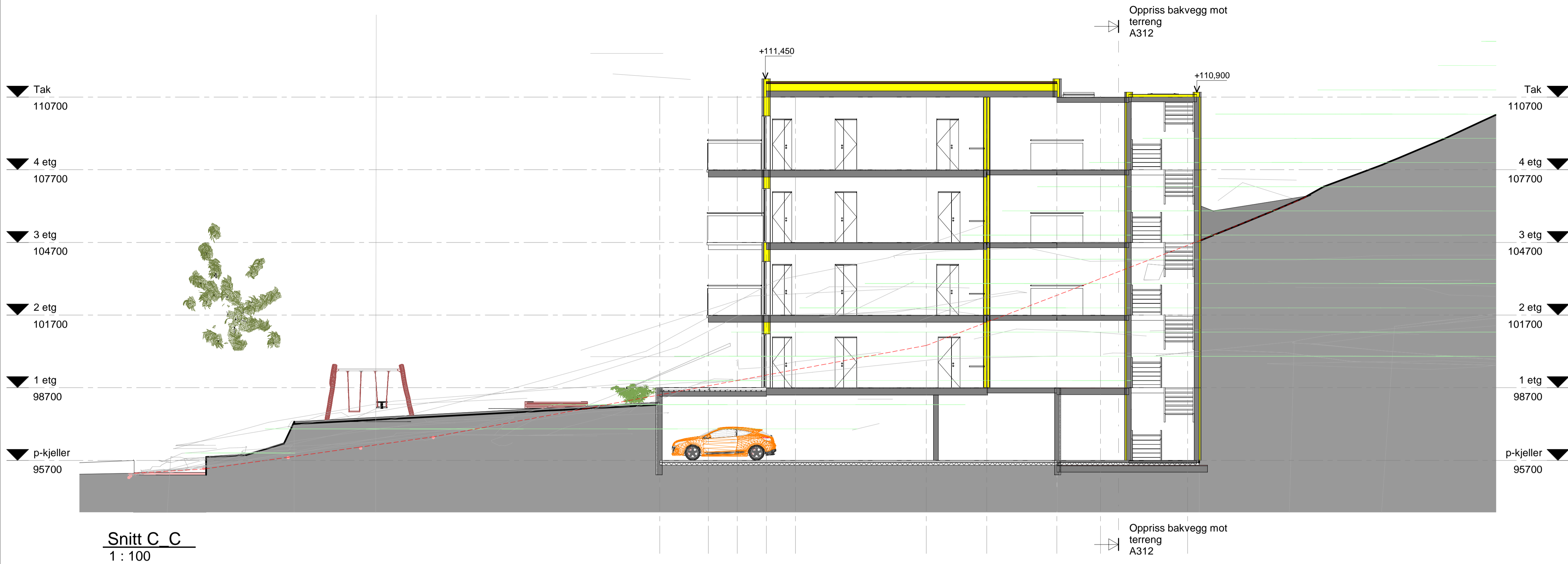
-svalganger innv4etg_blokkB-C
