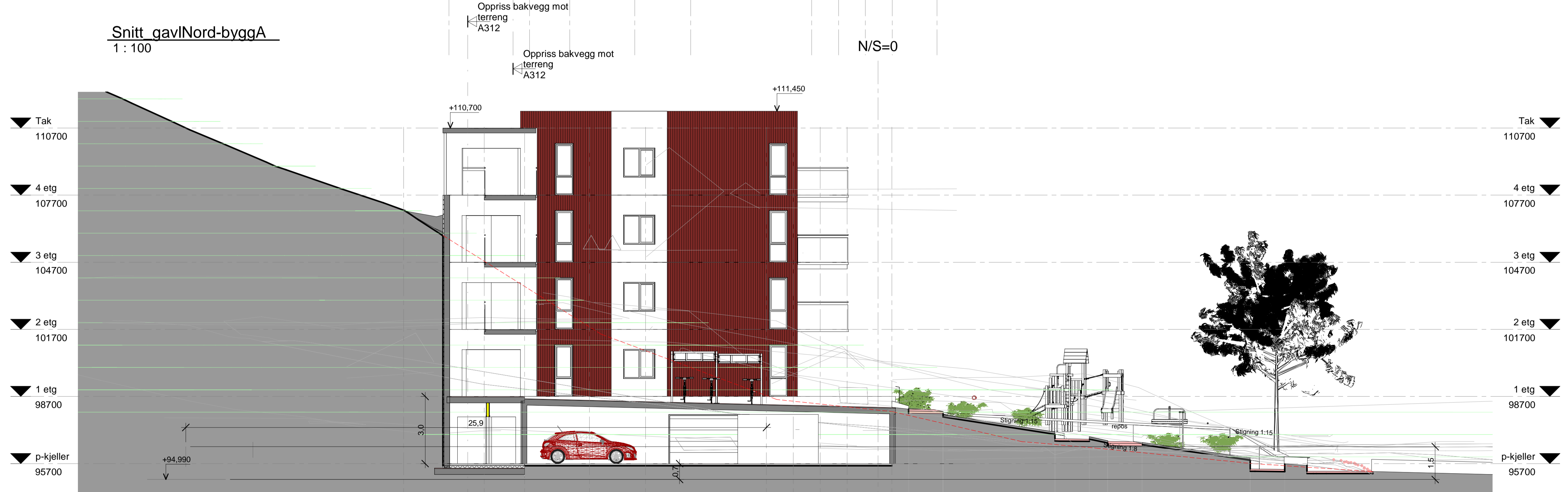
Snitt_gavlSør-byggB 1 : 100
