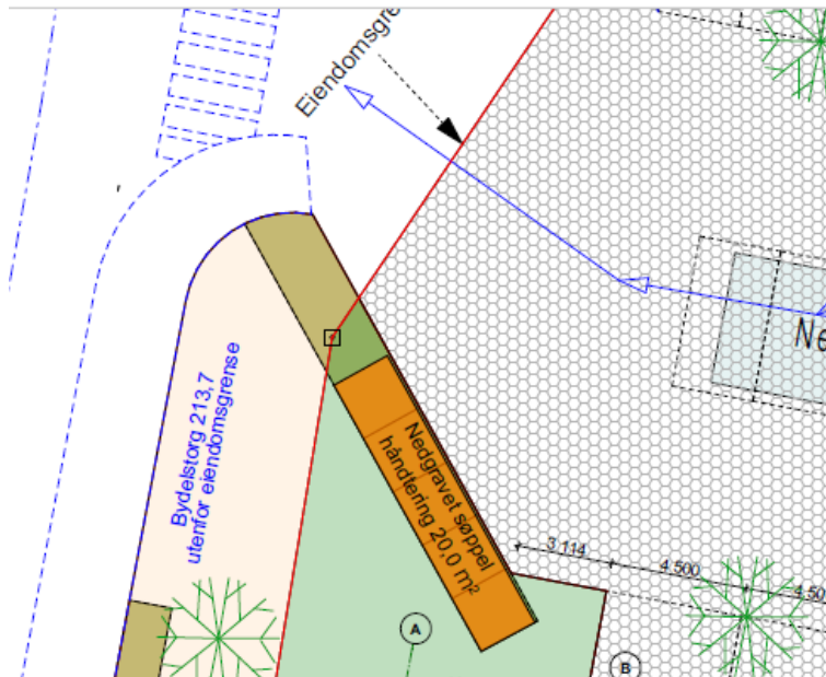
Nedgravd søppelløsning
