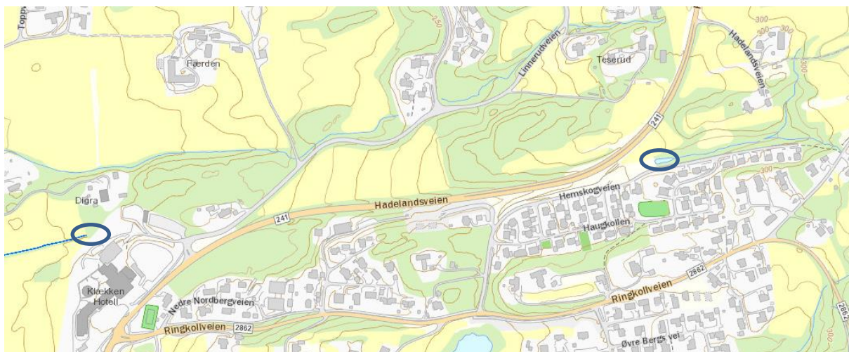
Figur 3: Innløp og utløp på OV800mm ledning er vist med blå ringer.
