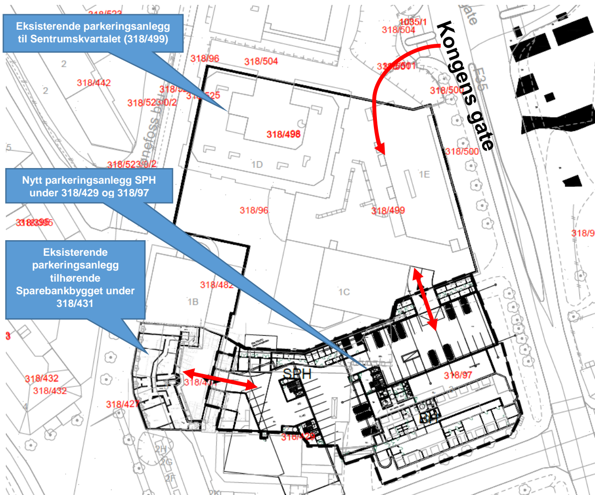
Figur 17 Illustrasjon som viser hvordan tilkomst til parkering er tenkt løst (under terreng).
