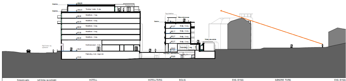
Figur 35 Prinsippnitt som viser siktlinj fra vestre ende av Søndre torv. BKB1 med 5 etasjer.
