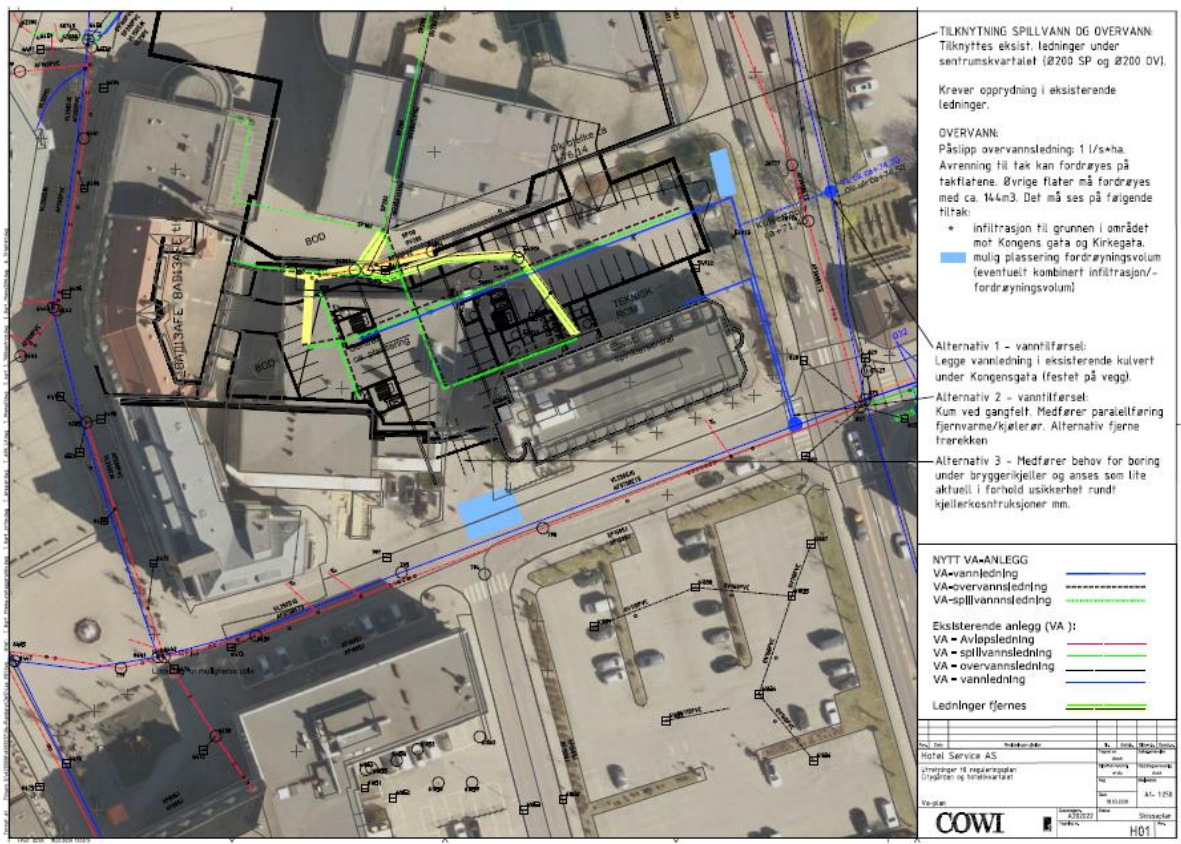
Figur 23 Utdrag fra rapporten Teknisk infrastruktur - vann og avløp for teknisk plan, som ligger ved planforslaget
